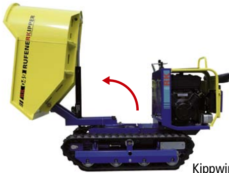
Kippwinkel 90° Fahrwerk mit Pendelrollen
